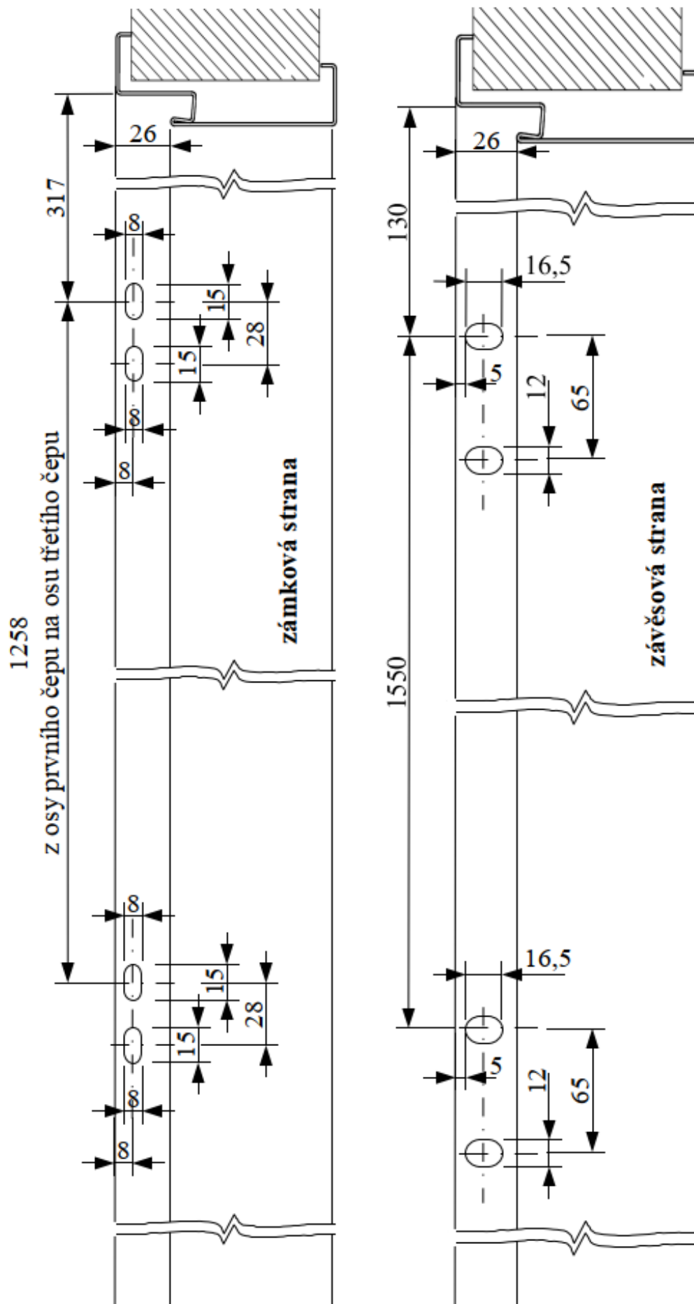
Obr. 1 rozměry otvorů pro bezpečnostní prvky dveří DPB 2
